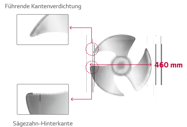
Lüfter Typ 2
