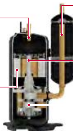
Inverter Doppelrollkolbenverdichter
