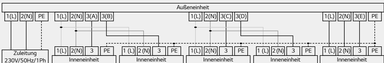
Schaltplan
